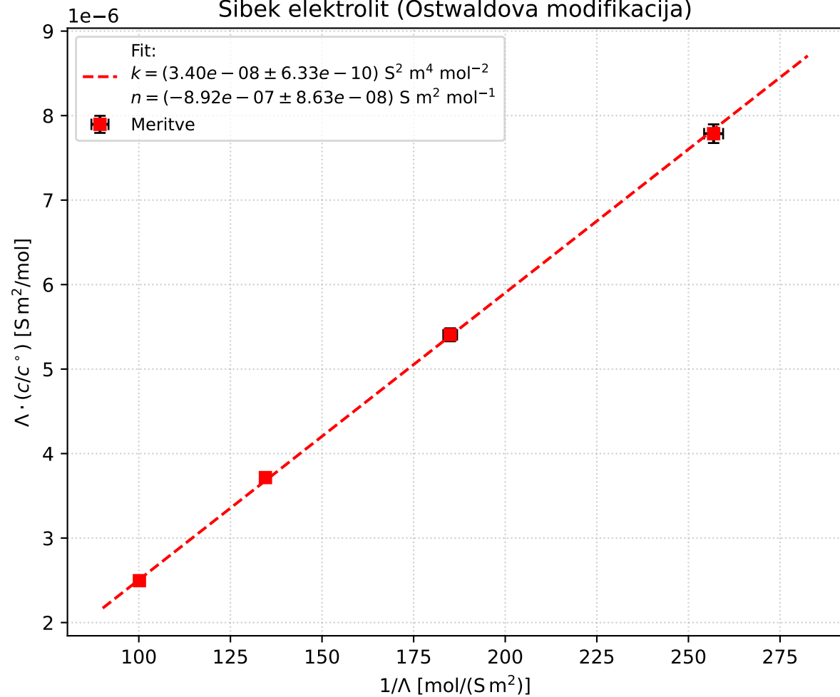
Šibek elektrolit (Ostwaldova modifikacija)
