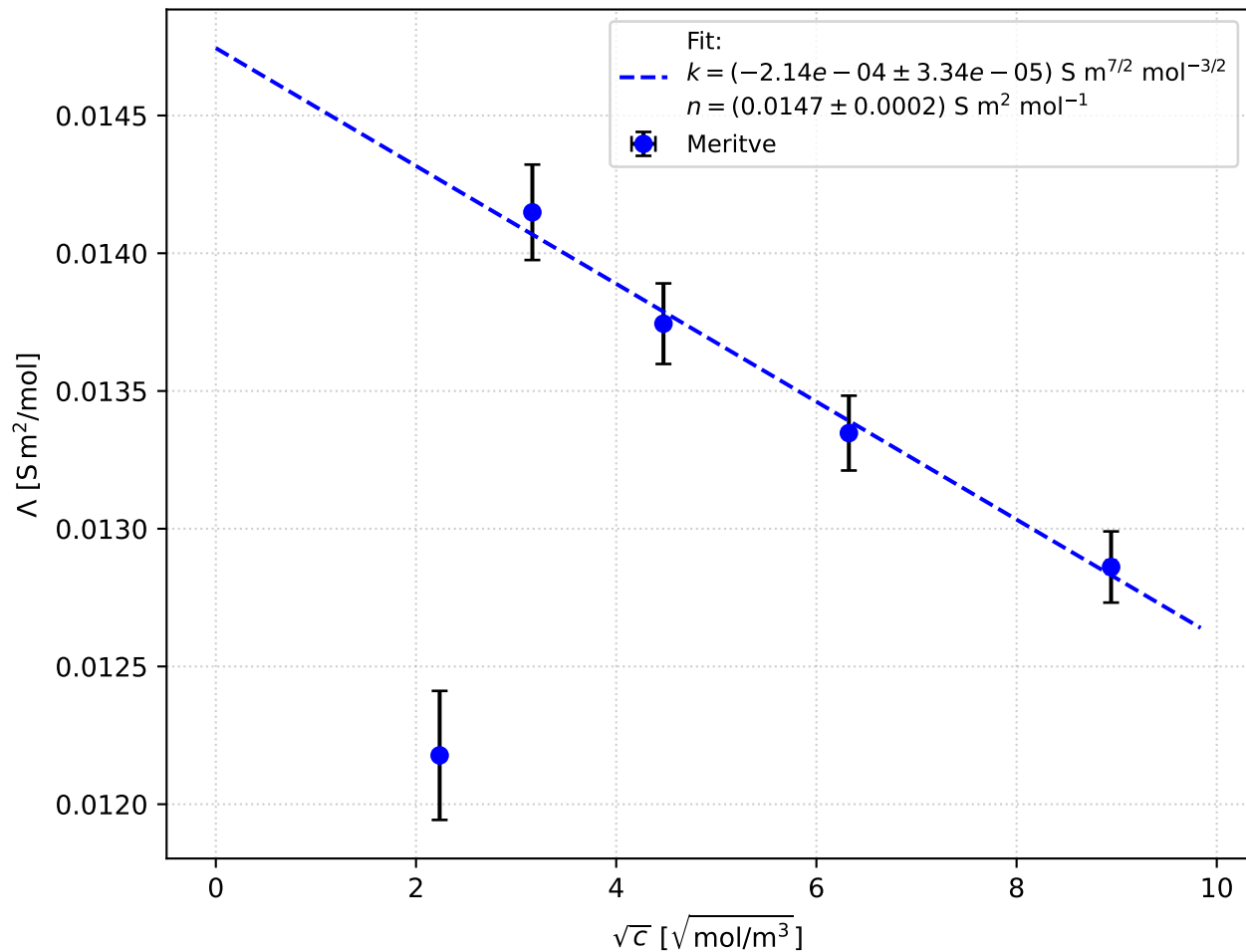
Močan elektrolit (Kohlrauschov zakon)
